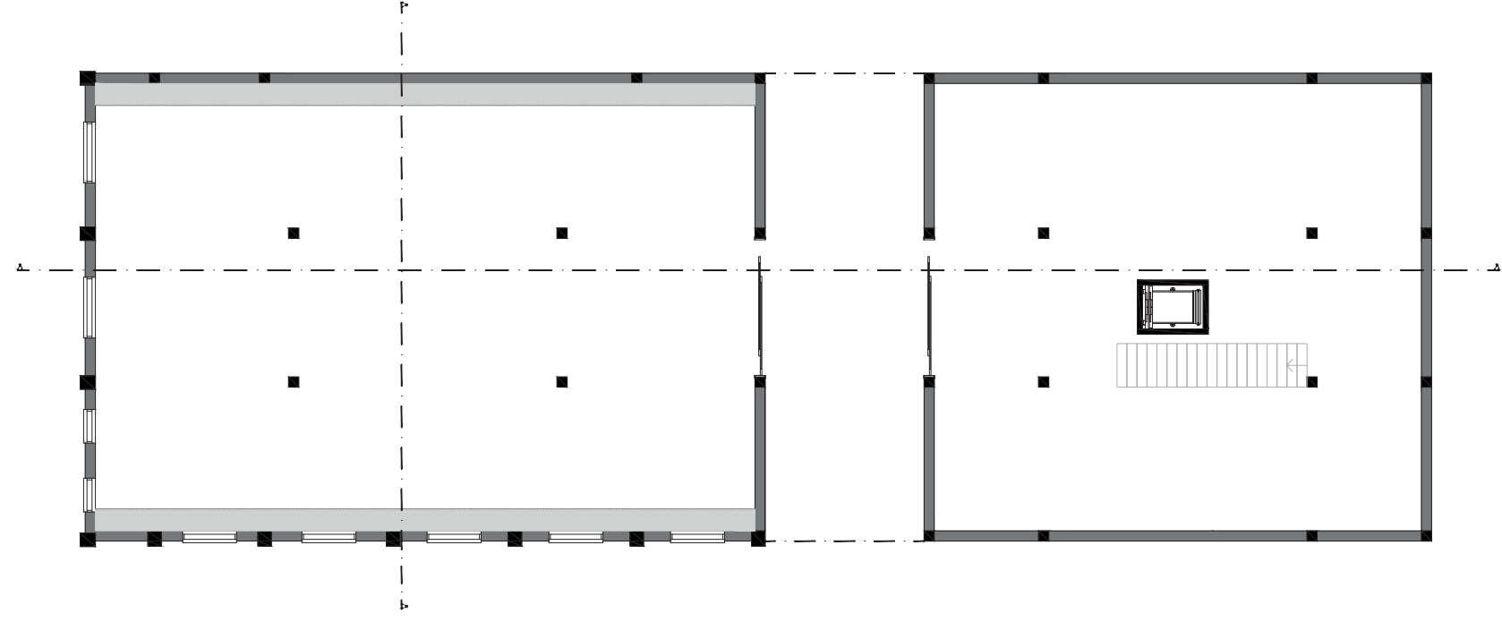
PLANTA 4o ANDAR ESCALA 1:200
